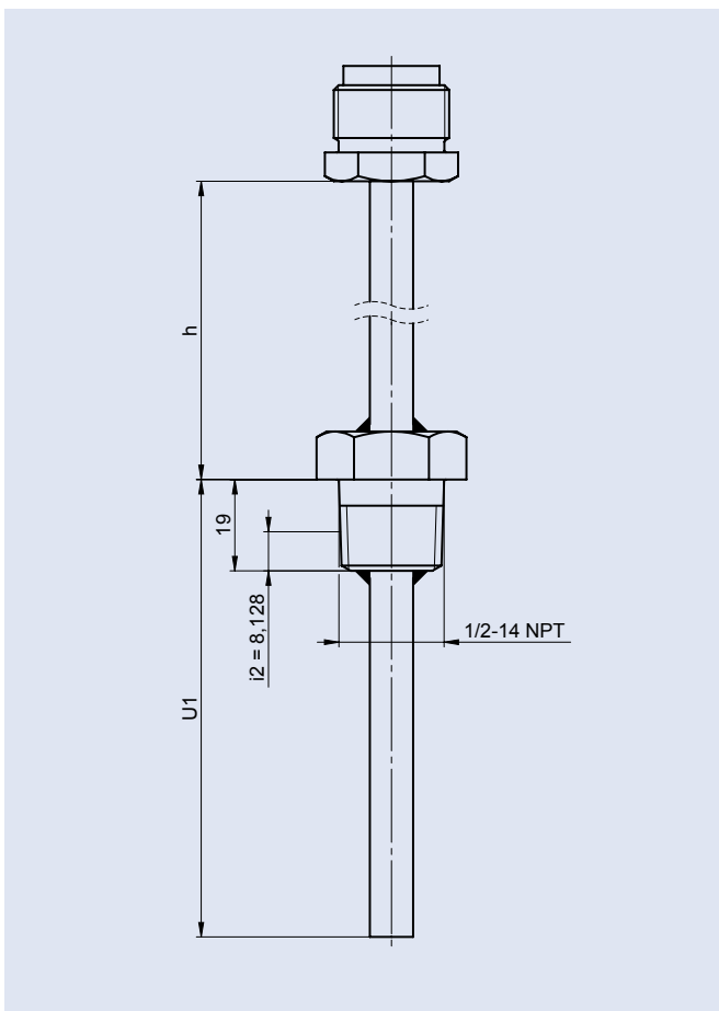
Schutzrohr mit \frac{1}{2} " NPT-Gewinde
