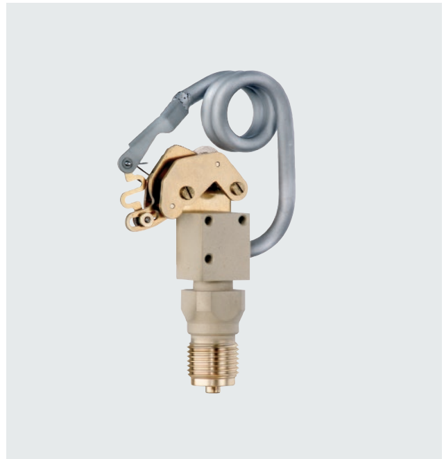
Rohrfeder-Messsystem in Schraubenform
